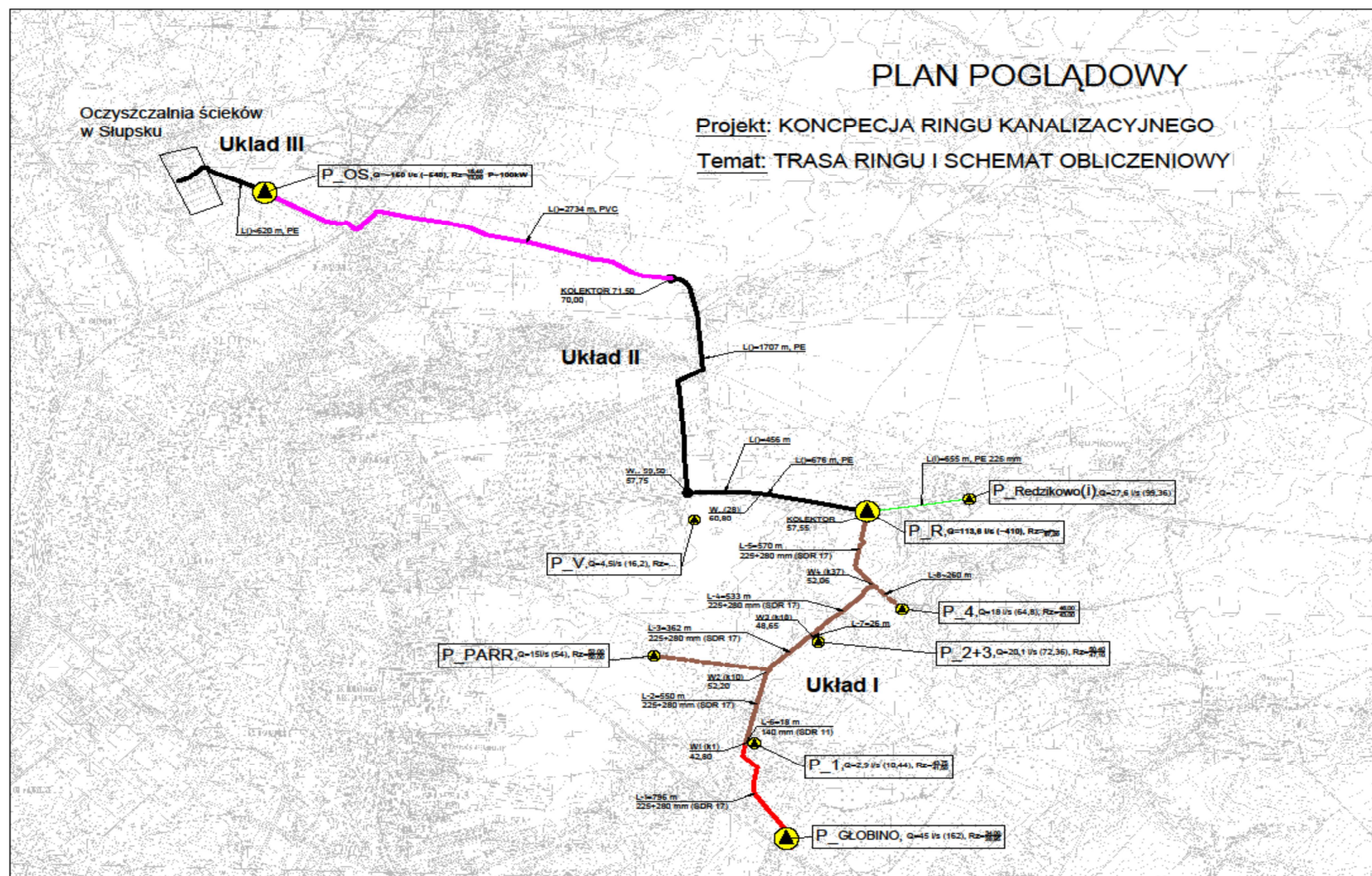
Rysunek 3 - Schemat hydrauliczny planowanego Ringu kanalizacyjnego
